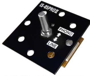
VESTAX IS-05PRO II INPUT SWITCH
