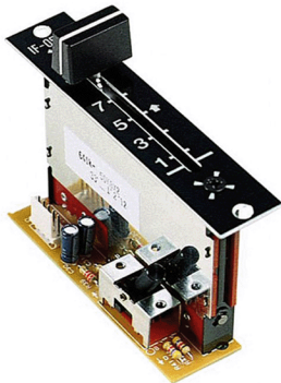
IF-07PCV INPUT VOLUME FADER
