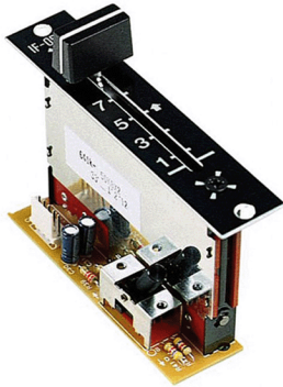
VESTAX IF-05PCV INPUT VOLUME FADER
